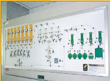
► EN Electric control board with synoptic panel SL Pregledna električna plošča HR Pregledna električna ploča PL Szafa elektryczna z ekranem synoptycznym RU Электрический щит с мнемосхемой ZH 帶示意圖符的控制櫃
